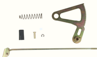
Reparo da Alavanca de Freio de Mão Renault Traffic/GM Space Van
